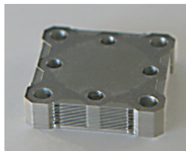
Mikrowärmetauscher aus 1.4301
