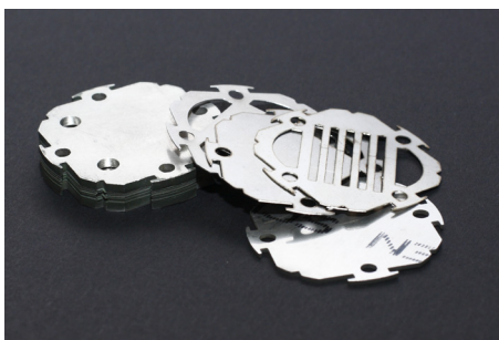
Mikrowärmetauscher aus 1.4301
